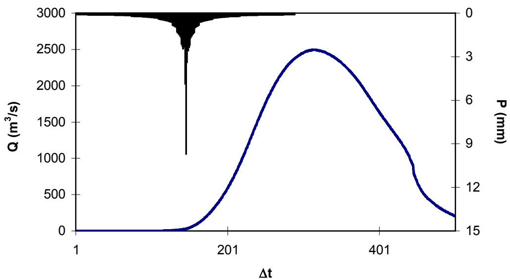
FIGURA 2.5 – HIDROGRAMA TOTAL AFLUENTE AO RIACHO DO MEIO (TR = 10000 ANOS)
