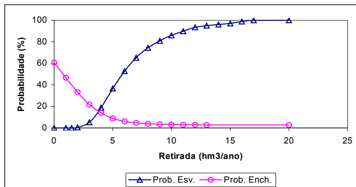
FIGURA 2.9 – PROBABILIDADES DE Esvaziamento e Enchimento
