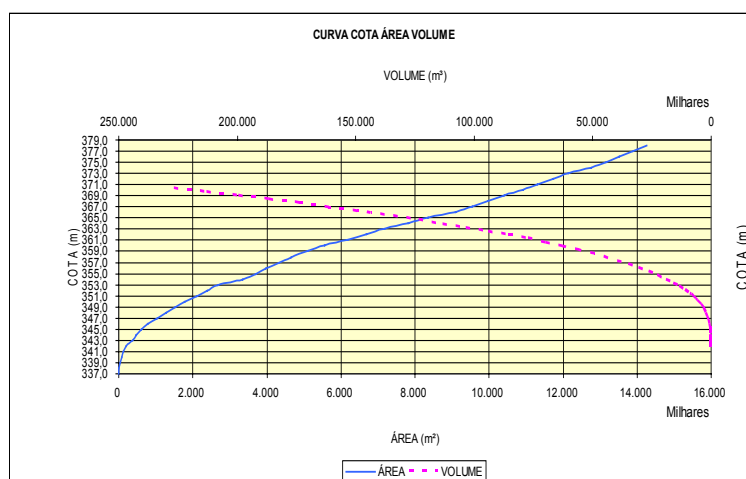
FIGURA 2.8 – CURVA COTA – ÁREA – VOLUME
