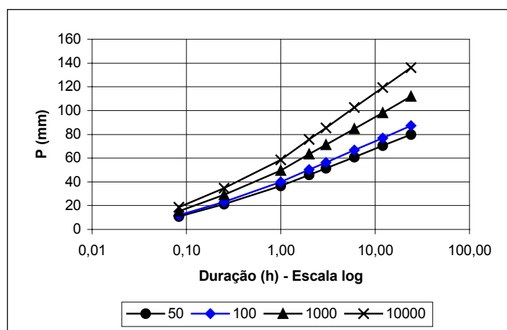
FIGURA 2.3 – CURVAS INTENSIDADE-DURAÇÃO-FREQÜÊNCIA
